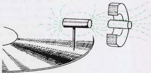
Fig. 8 Principe van een groeftaster
